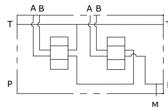
ESQUEMA HIDRÁULICO
