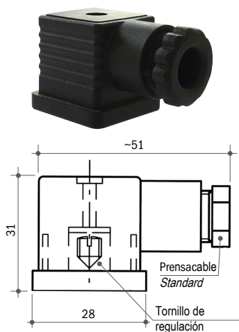
Conector DIN 40050
