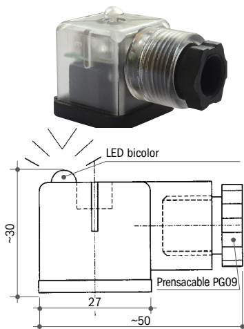
Conector transparente con Led bicolor rojo/verde Tipo CLB
